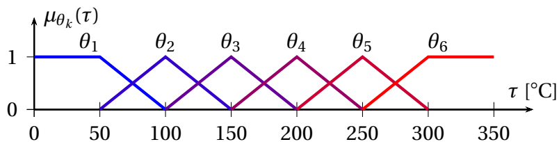
Figura 3.1: Partición difusa de la temperatura en el reactor.
